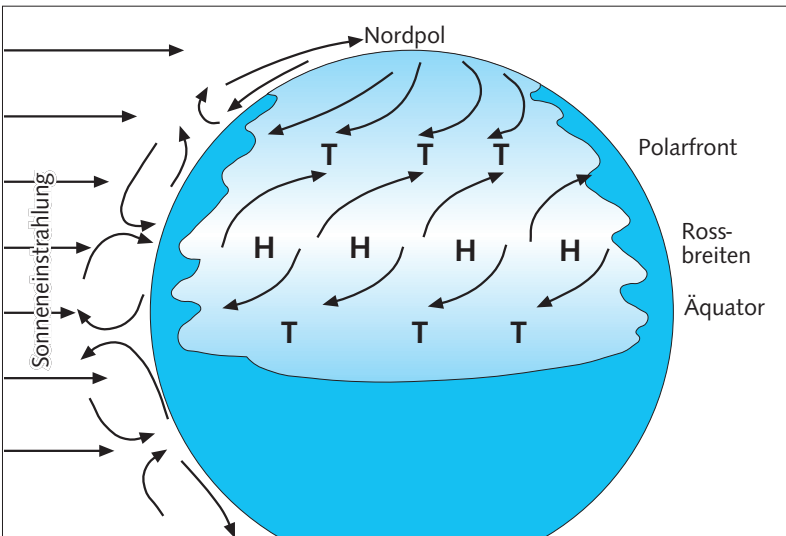
2/2: Das planetarische Windsystem.
