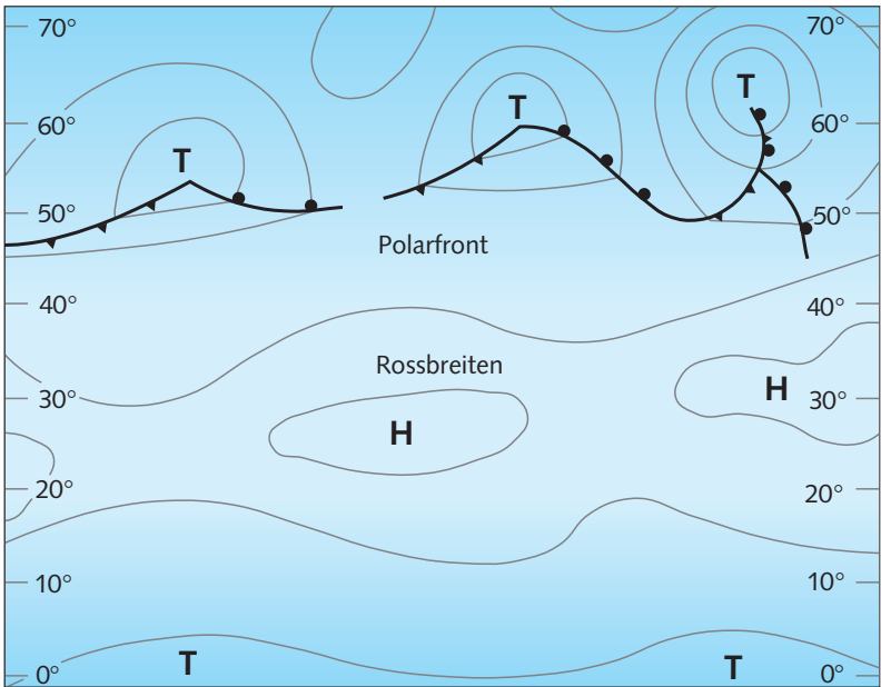
2/3: Typische Druckverteilung mit erkennbaren Gürteln des planetarischen Windsystems.
